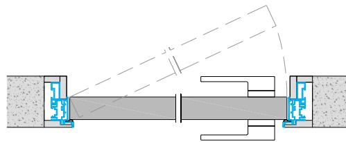
Открытие «в проем» Push opening
