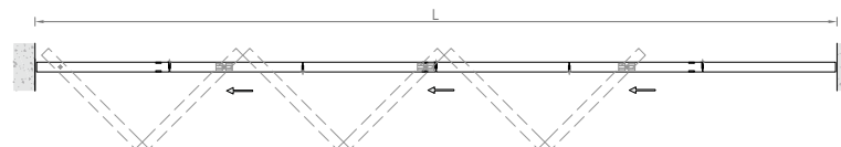
Перегородка TRANSFORMER, модель Vario. N - Количество полотен, складывающихся в одну сторону. L max = 5800 mm, H max = 3000 mm TRANSFORMER partition, Vario model. N - Number of leaves folding to one side. L max = 5800 mm
