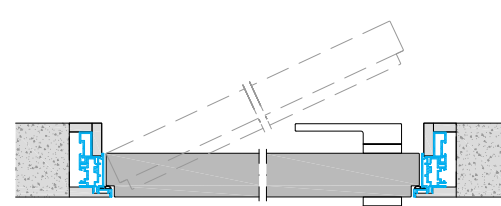
Открытие «в проем» - компланарность Push opening. Complarity
