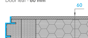
Полотно Alu - 60 mm Alu door leaf - 60 mm
