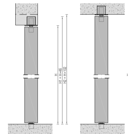
Дверь в проеме Door in the wall-opening
