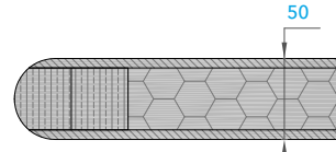
Полотно TONDA - 50 mm TONDA door leaf - 50 mm
