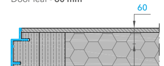
Полотно Alu - 60 mm Alu door leaf - 60 mm
