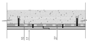
Продольное соединение Longitudinal connection
