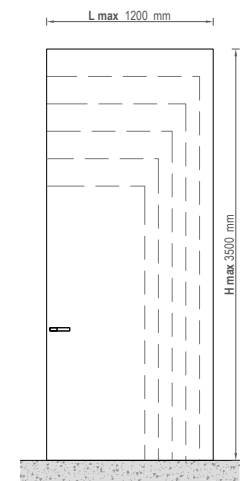
Максимальные размеры Maximum dimensions
