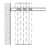
Перегородка TRANSFORMER, модель Vario. N - Количество полотен, складывающихся в одну сторону. L max = 5800 mm, H max = 3000 mm TRANSFORMER partition, Vario model. N - Number of leaves folding to one side. L max = 5800 mm
