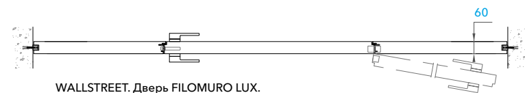
WALLSTREET. Дверь FILOMURO LUX. WALLSTREET and FILOMURO LUX door
