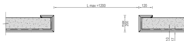
Обрамление проема Framing of the opening
