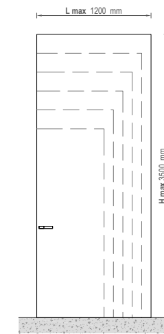
Максимальные размеры Maximum dimensions
