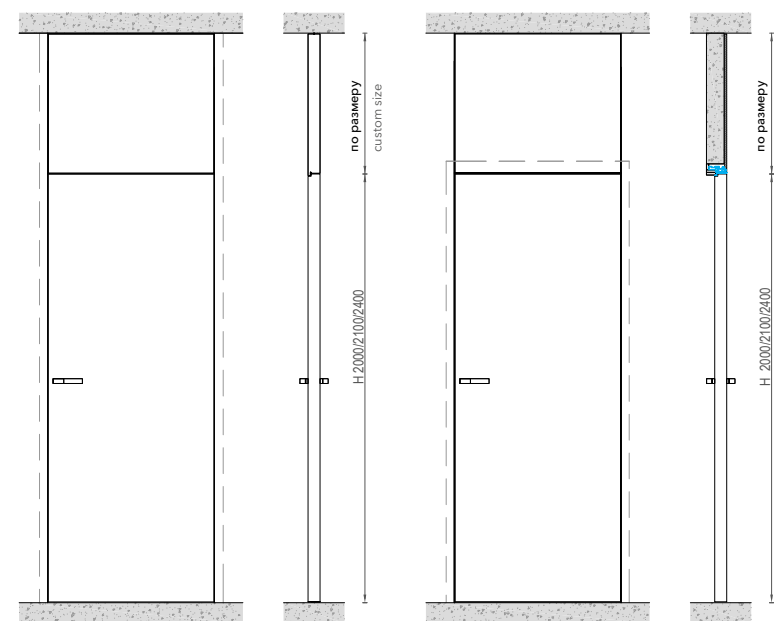
Тип В. Дверь с фрамугой «под потолок». Короб без перемычки. Invisible door with transom panel Type B.
