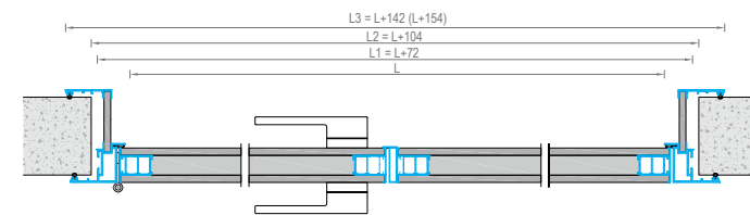
Двустворчатая дверь Double door
