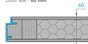
Полотно 60 mm с алюминиевой кромкой Door leaf with aluminium edge - 60 mm
