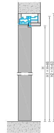
Открытие "из проема" - компланарность Pull opening. Complanarity
