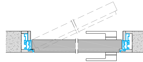
Открытие «в проем» - компланарность Push opening. Complanarity
