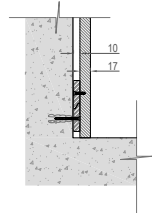
Вертикальное сечение Vertical cross-section
