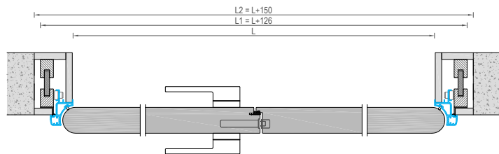
Двустворчатая дверь Double door
