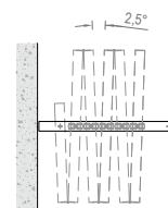
Перегородка TRANSFORMER, модель Medio. Без нижнего направляющего канала. N - Количество полотен, складывающихся в одну сторону. L max = 5800 mm, H max = 3000 mm TRANSFORMER partition, Medio model. Without floor track. N - The number of leaves that can be folded in one direction L max = 5800 mm, H max = 3000 mm
