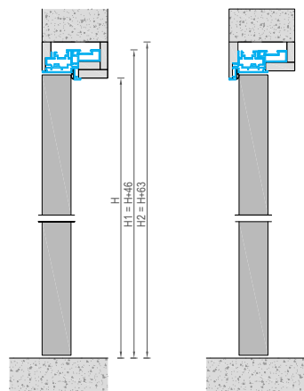
Открытие «из проема» - компланарность Pull opening. Complanarity
