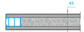
Полотно UNIX - 45 mm UNIX door leaf - 45 mm
