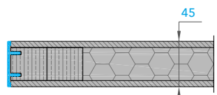
Полотно Alu - 45 mm Alu door leaf - 45 mm
