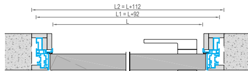
Открытие "из проема" - компланарность Pull opening. Complarity
