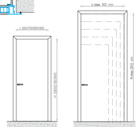
Стандартные размеры (условные) Standard dimentions (indicative)
