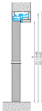
Открытие "из проема" - компланарность Pull opening. Complanarity
