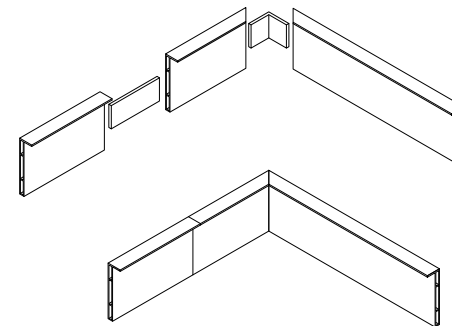
Соединительные элементы плинтуса Plinth connectors
