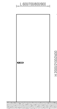
Стандартные размеры (условные) Standart dimitions (indicative)
